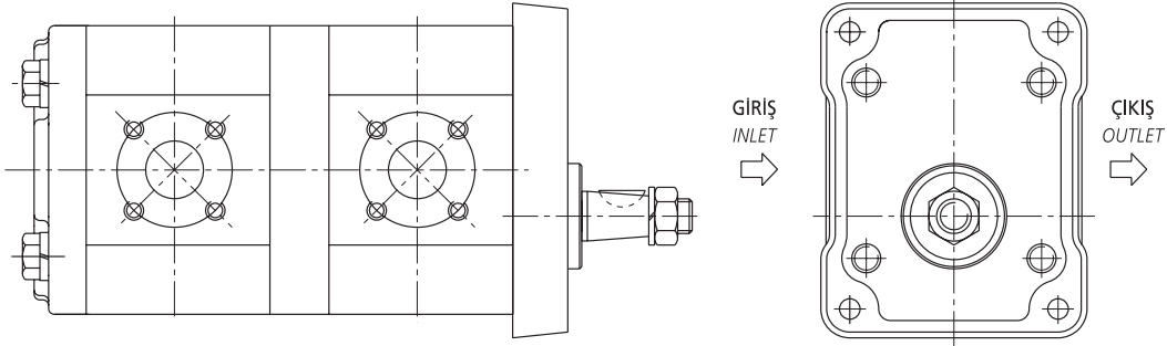
Şekil 4. Pompa Dönüş Yönü
