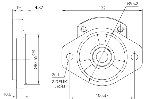
G KAPAK TİPİ / Flange type
